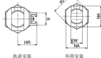
轨道安装
