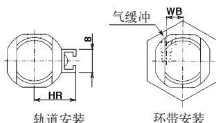
轨道安装
