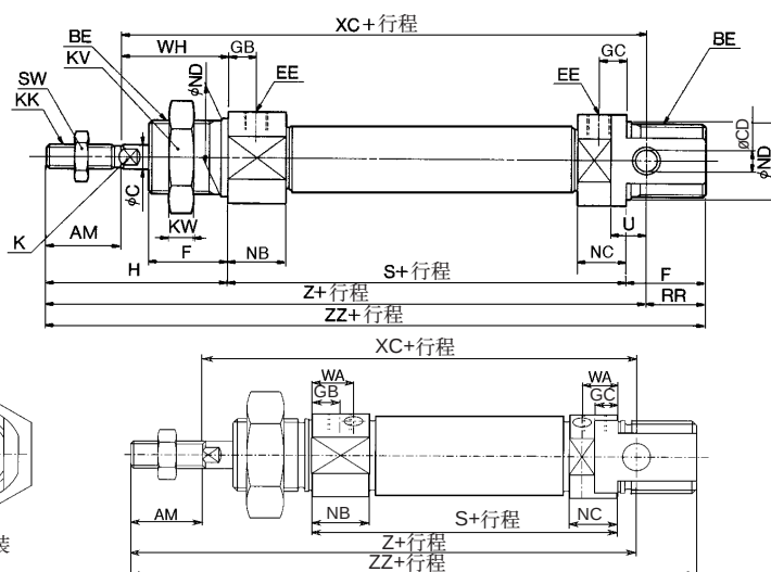
环带安装
