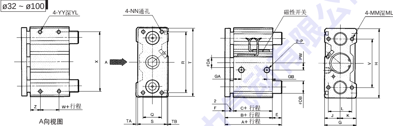
MGQM (滑动轴承)
