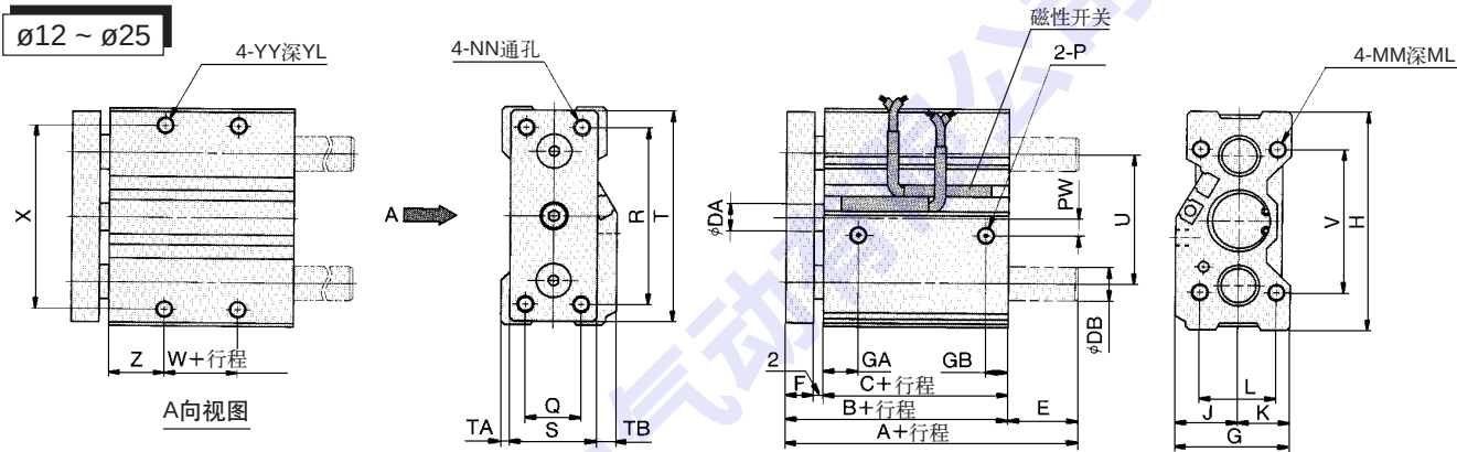
MGQM (滑动轴承)
