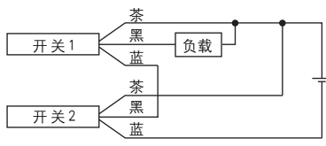
2线式的场合·2个OR连接
