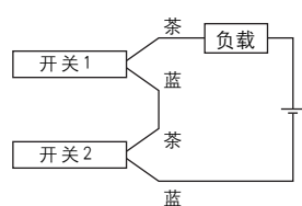
2线式的场合·2个AND连接
