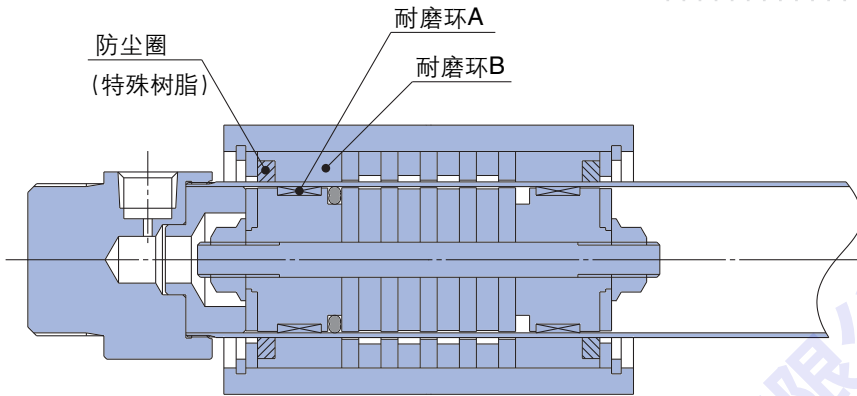
■ CY3B系列 ■
