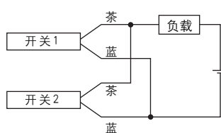
2线式的场合·2个OR连接
