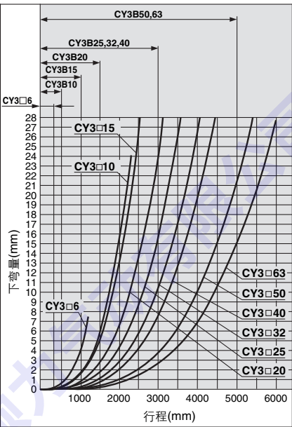
※图示下弯量为外部滑动部分运动到行程中间时的值
